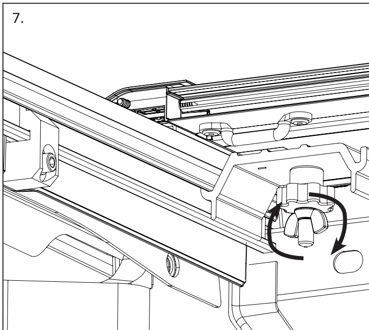
Tighten tie-down (TD) | Apriete el gancho | Attachez l'ancre
