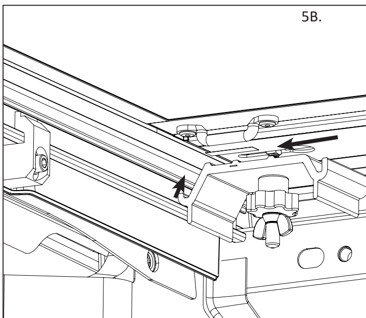
Install tie-down (TD) | Instalar gancho | Installer l'ancrage
