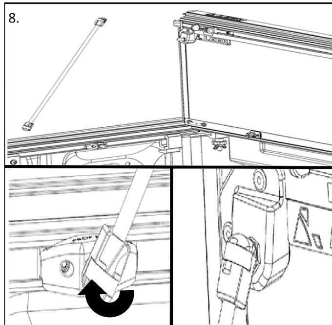
Install prop rod (PR) | Instalar varilla de apoyo | Installer la tige de prop
