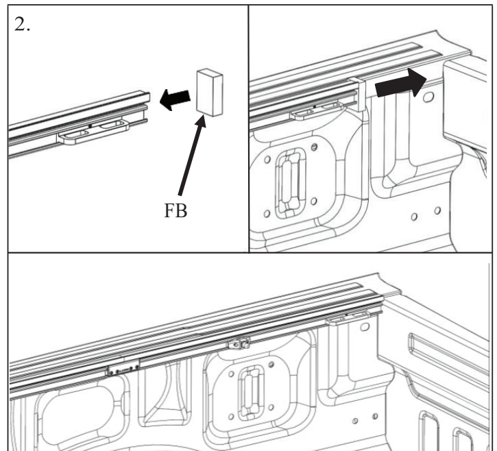
2. Push forward to bulkhead (LR, RR, FB) | Empuje hacia el mamparo | Pousser contre le mur
